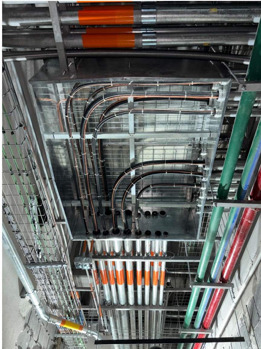
ALIMENTADORES GENERALES EN REMODELACIÓN DE TIENDA
